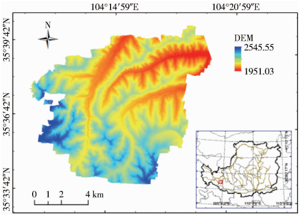
图2 甘肃省榆中县龙泉乡 DEM 及所在黄土高原位置图 Fig.2 DEM and location of study area
