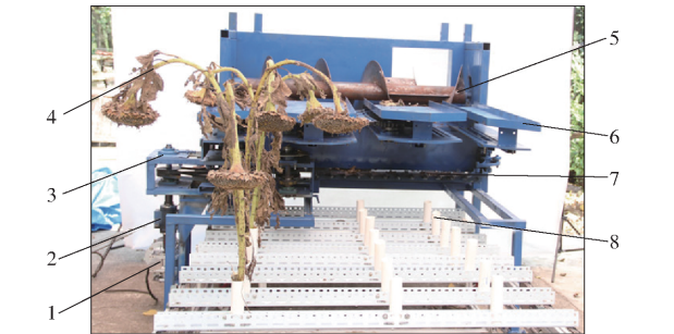
图 7 试验台架
