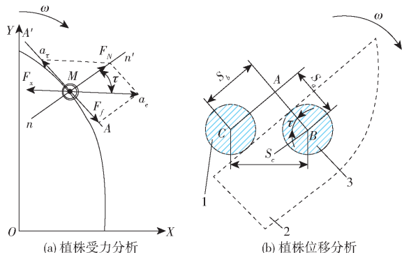
图4 植株受力及位移分析图
