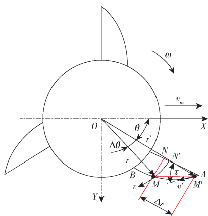
图3 静态滑切角恒定刀刃切割器结构示意图
