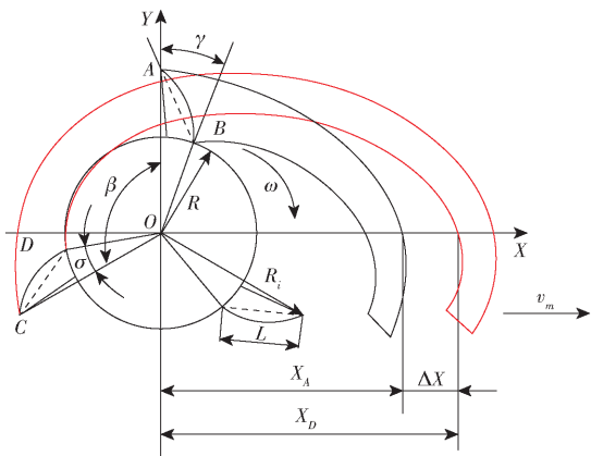
图5 割刀运动轨迹
