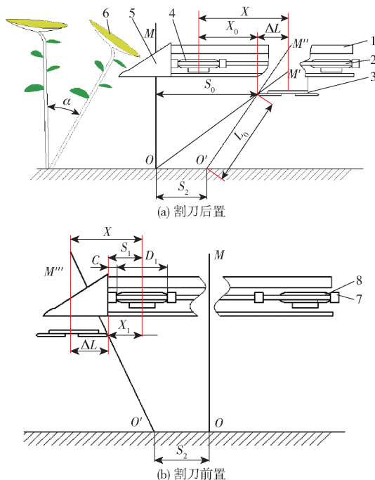
图6 夹持切割几何示意图
