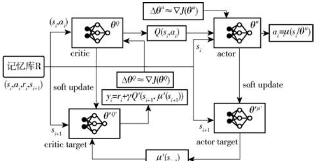
图 1 DDPG 算法网络结构图
