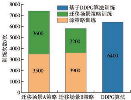
图 13 混杂障碍场景下收敛所需迭代次数
