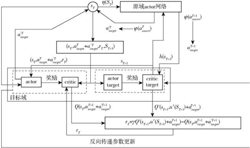
图 5 基于迁移学习的 DDPG 算法参数更新示意图
