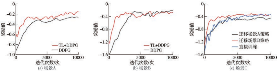
图12 不同场景下训练时的奖励值变化曲线
