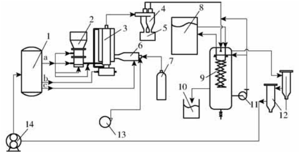
图 1 热裂解装置工艺流程图
