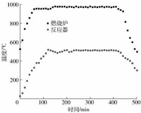
图 7 一个试验周期内燃烧炉和反应器的温度分布
