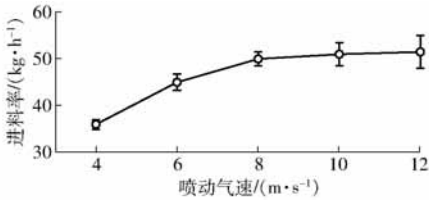
图 5 喷动气速对进料率的影响
