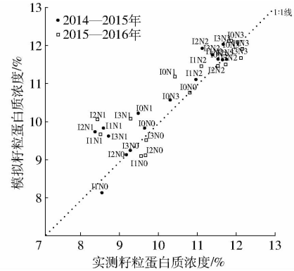
图2 2014—2016年16种不同水肥处理下籽粒蛋白质浓度模拟值与实测值对比
