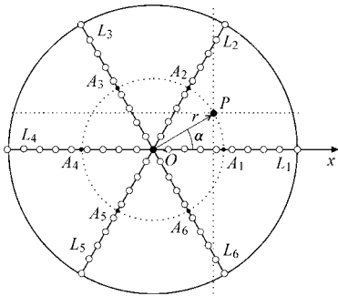
图 3 两次插值方法示意图
