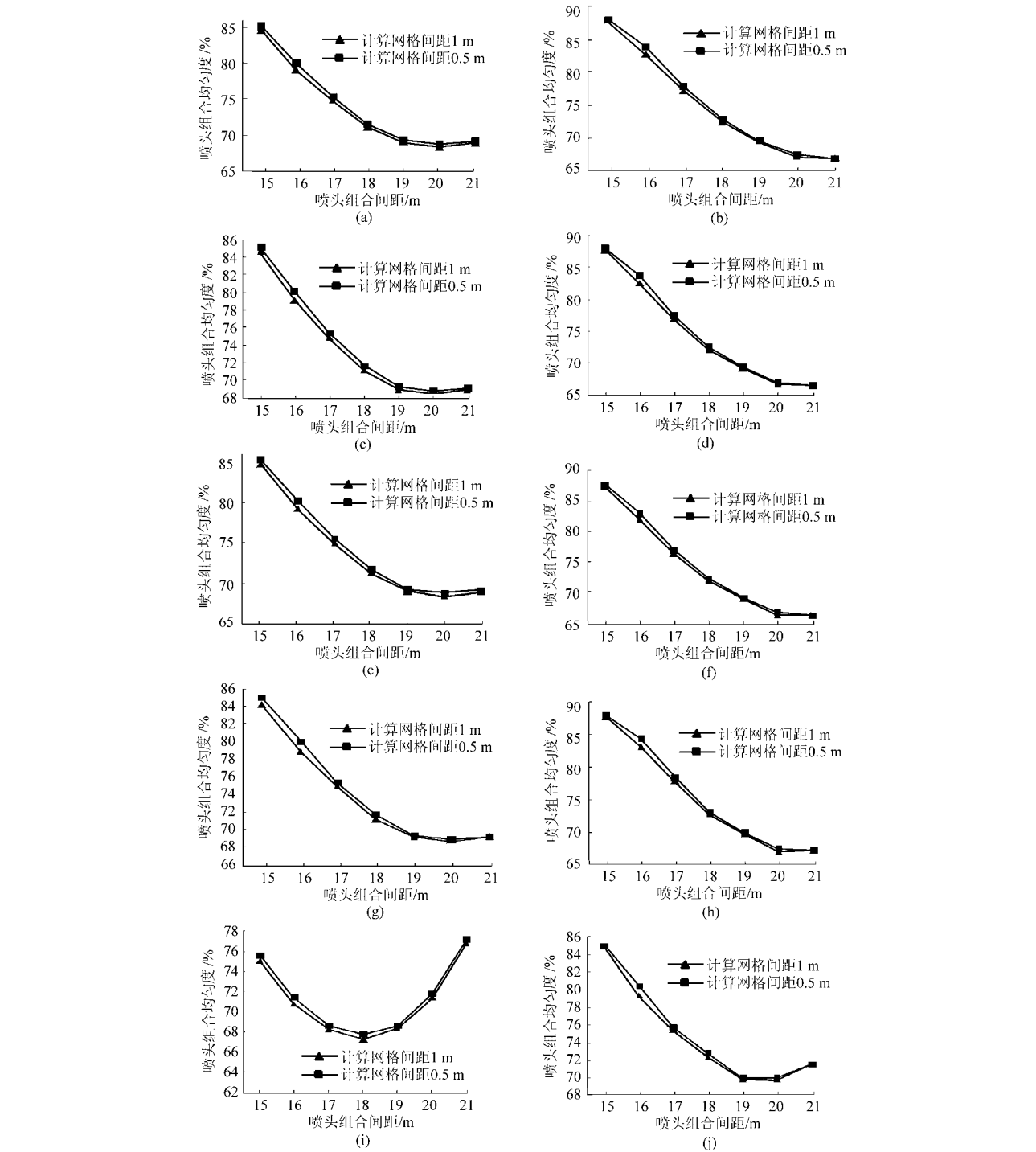
图 8 不同计算网格点间距的喷头组合均匀度
