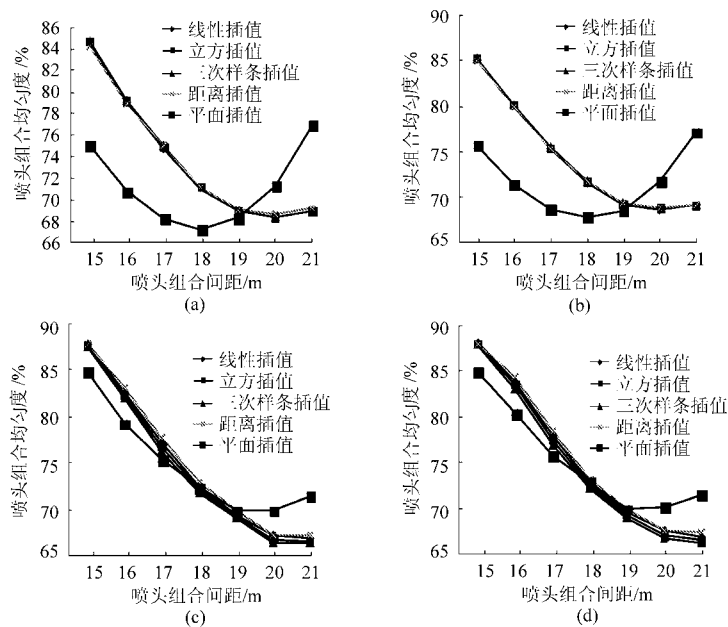
图 6 不同插值方法下喷头组合均匀度随组合间距的变化曲线
