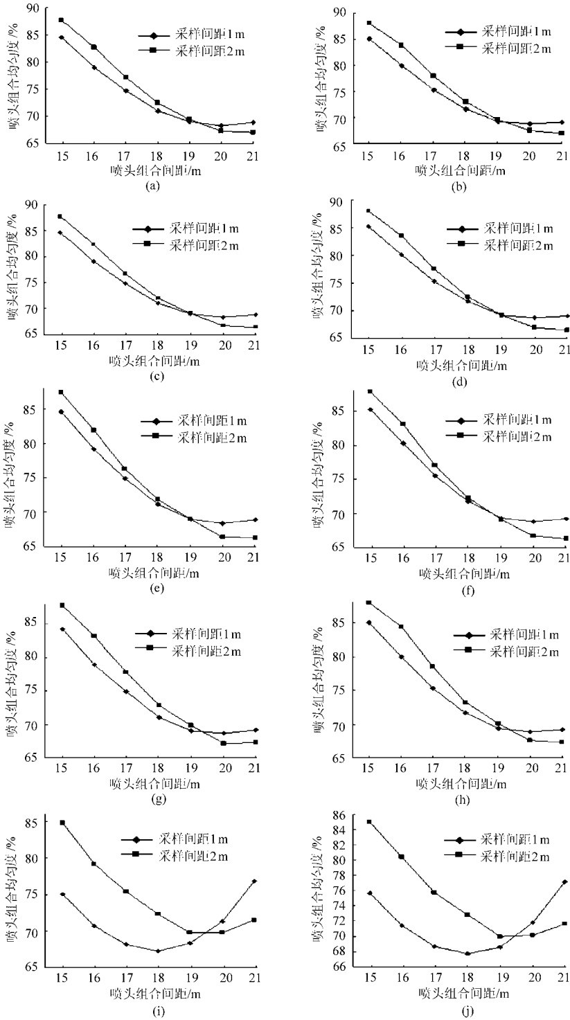
图 7 不同采样间距的喷头组合均匀度
