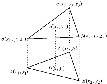
图 5 平面插值方法示意图
