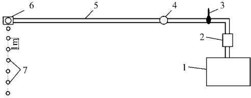
图 1 喷灌试验设备布置示意图 Fig. 1 Sprinkler test equipment layout
