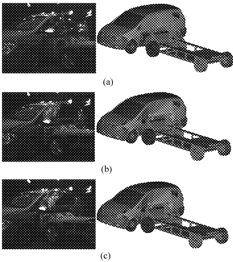
图 8 侧面碰撞整车变形时间历程 Fig. 8 Deformation of car in side impact (a) 第 20 ms (b) 第 60 ms (c) 第 100 ms
