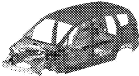
图 2 白车身有限元分析模型
