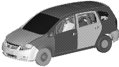
图 1 整车有限元模型
