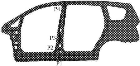
图 5 侧面碰撞车体侵入量测量点示意图 Fig. 5 Test points of intrusion displacement of body in side impact
